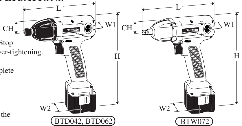
Dimensions : mm ( " )
