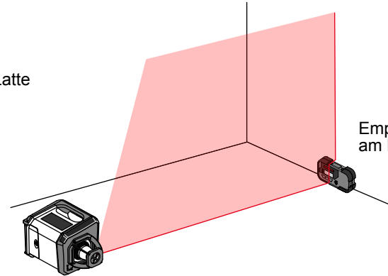
Laser in liegender Position
