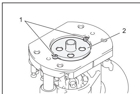
► 1. Screw 2. Template guide
