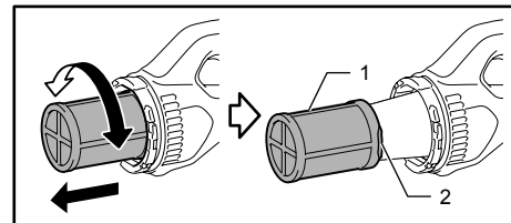
1. Préfiltre 2. Rebord de fixation
